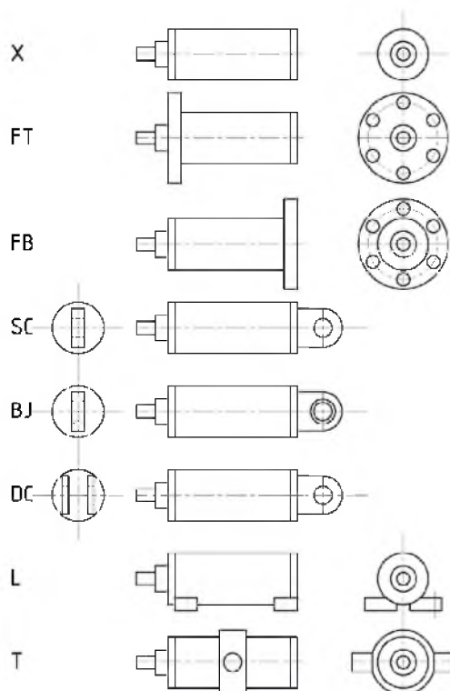
ТИПЫ КРЕПЛЕНИЯ КОРПУСА ГЦ
