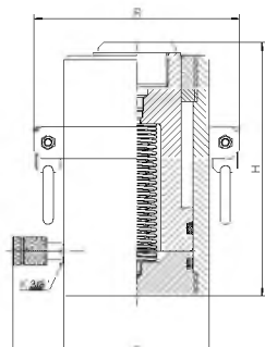
Грузовые с пружинным и гравитационным (принудительным) возвратом поршня 5-100 тс
