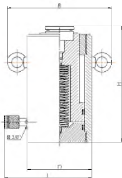
Грузовые с пружинным и гравитационным (принудительным) возвратом поршня 150-200 тс
