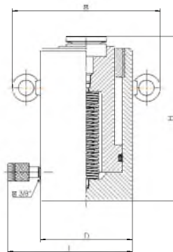
Грузовые с пружинным и гравитационным (принудительным) возвратом поршня 300-1000 тс
