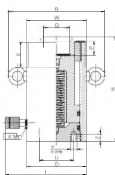
Домкраты универсальные с пружинным возвратом 150-200 т
