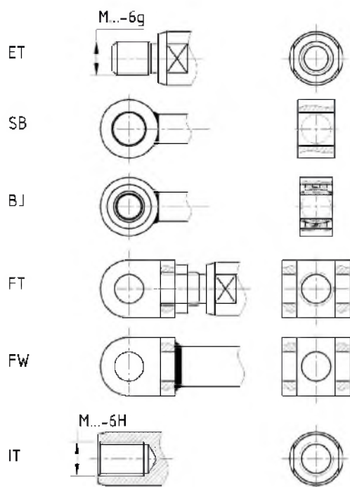
ТИПЫ КРЕПЛЕНИЯ ШТОКА ГЦ
